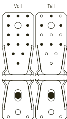
KR Langloch 135 mm 1101353L / 110135L
